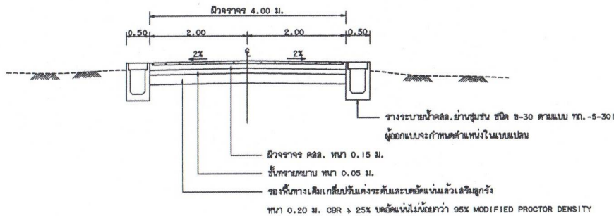
รูปตัดถนนคอนกรีตเสริมเหล็ก (กรณีจราจรระบายน้ำ)
